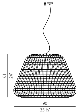
Esempio: versione con rosone IP20 Example: canopy version IP20
