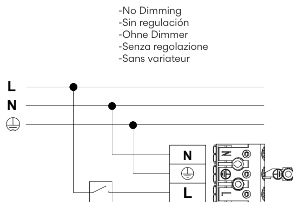
Diagram / Diagrama / Anschlusschema / Diagramma / Diagramme Z
